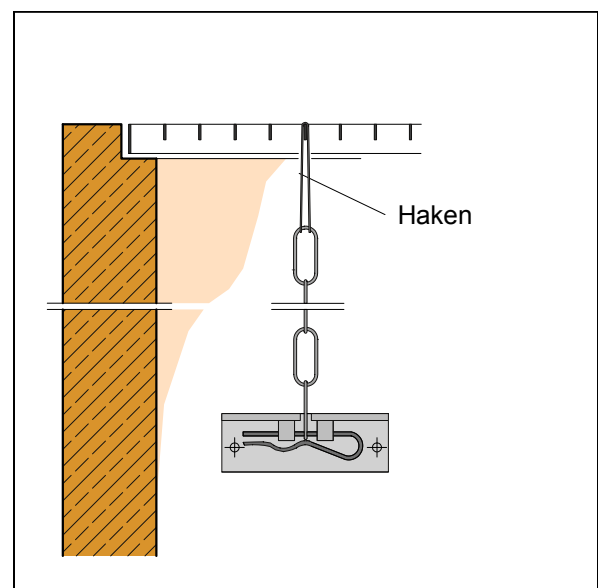
SONDER-GITTERROSTE-NOTAUSSTIEG
