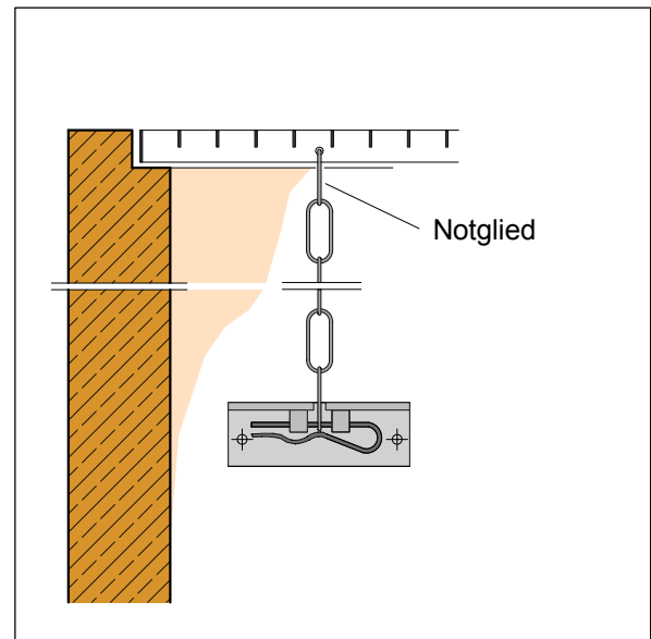
STANDARD-NOTAUSSTIEG
