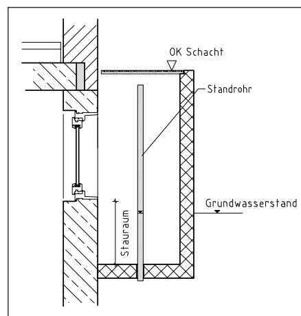
Standrohr
