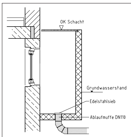
Ablaufmuffe DN110
