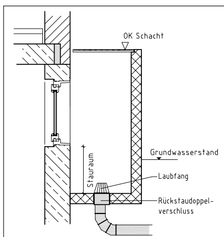
Rückstaudoppelschluss
